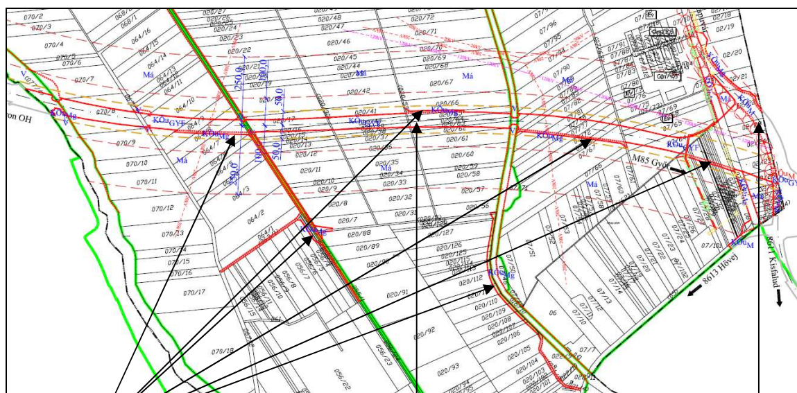
Kivonat a módosított szabályozási tervből
