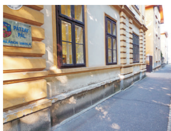
Reversion hálószonda a műkö lábazat felett a vakolati rétegek alatt elhelyezve → R-1
