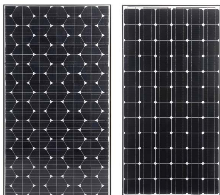
A kétféle HIT típusú napelem modul
